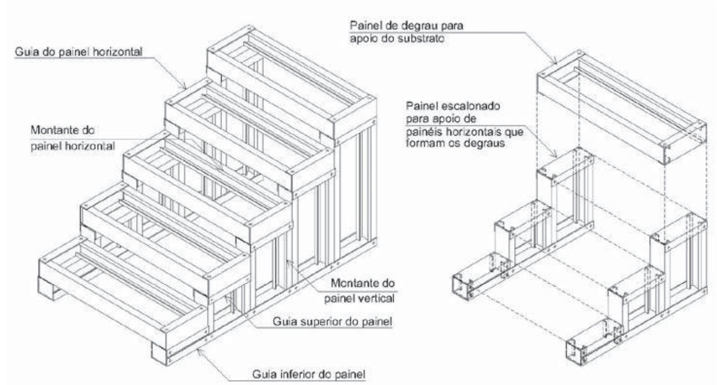
Figura 4.17 - Desenho esquemático de uma escada de painéis escalonados
