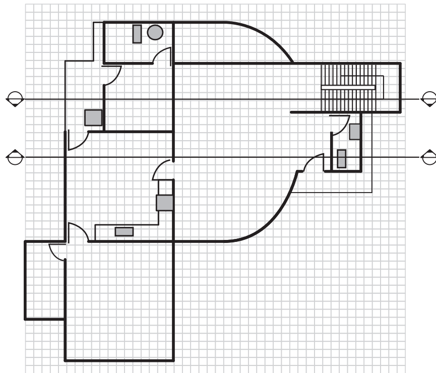
Figura 8.1 - Uso de malhas geométricas modulares para projetos de arquitetura em LSF
