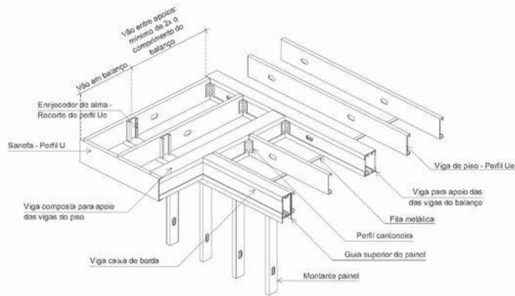
Figura 4.8 - Laje em balanço
