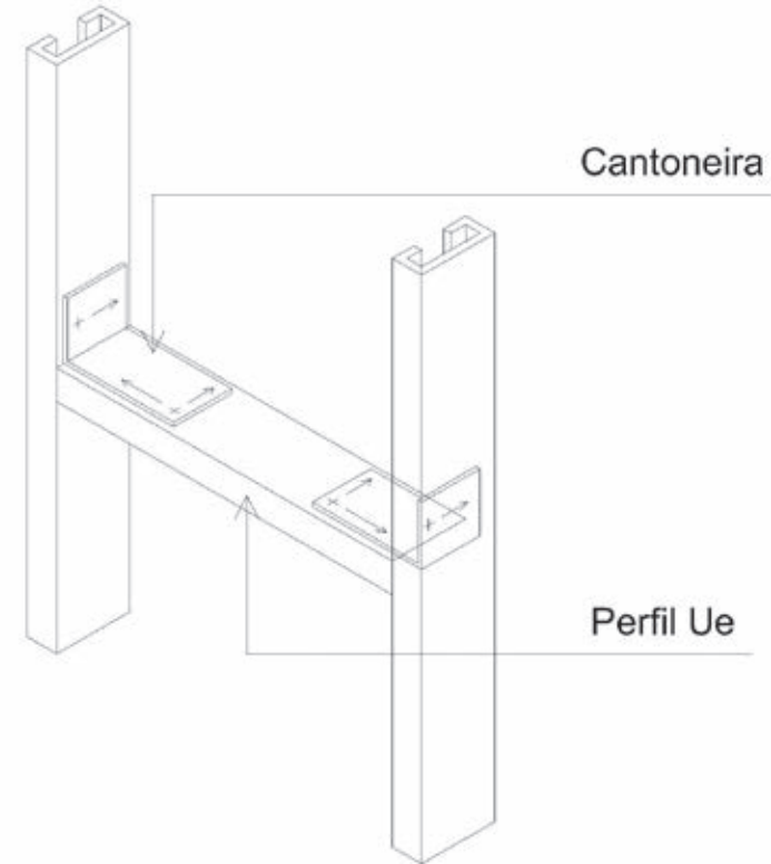
Figura 3.14 - Esquema de fixação de bloqueador através de cantoneiras
