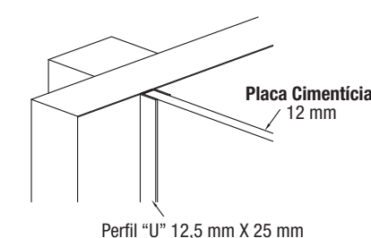
AMPLIAÇÃO 1
