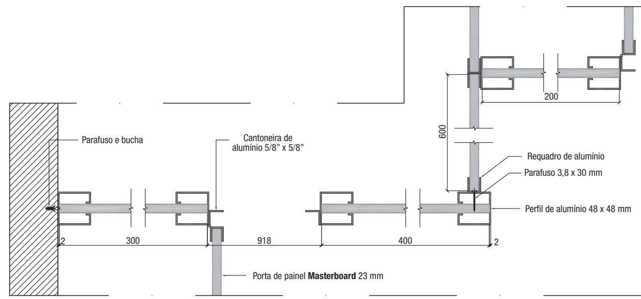
DETALHE 4
