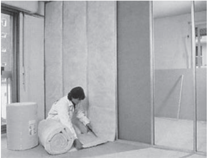
Foto 6.4 - Isolamento termoacústico (Fonte: Isover)
