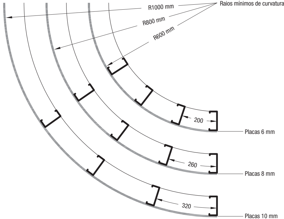
CORTE I-I PAREDES CURVAS
