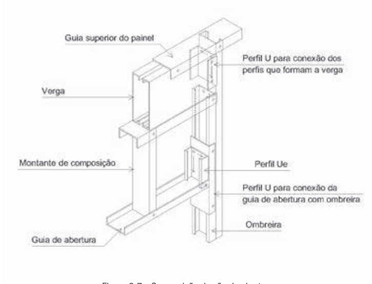
Figura 3.7 - Composição de vão de abertura
