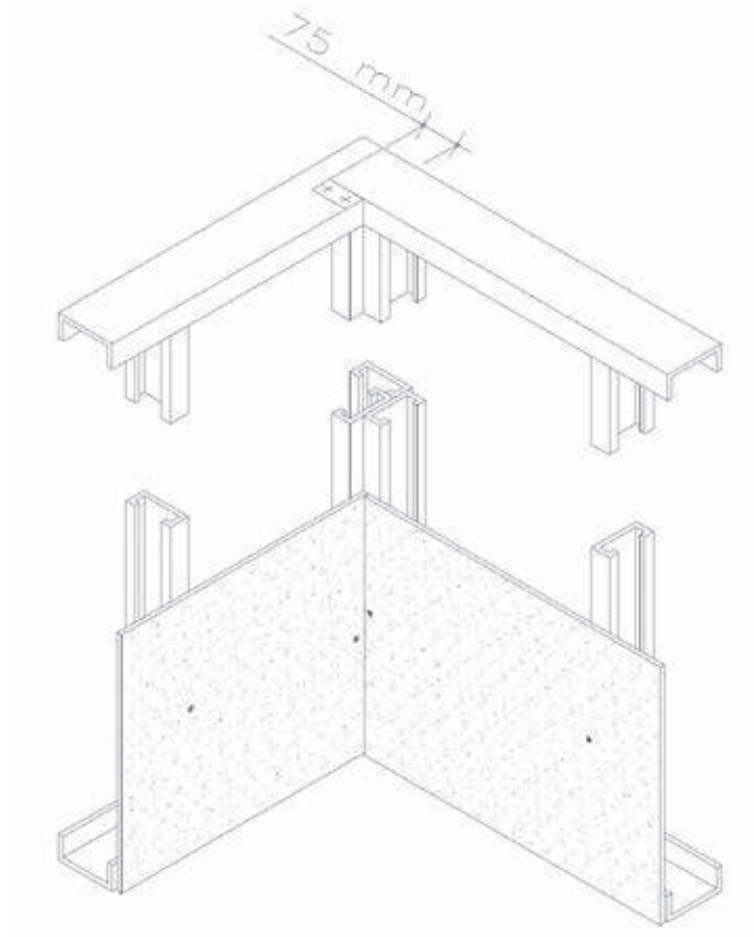
Figura 3.17 - Fixação de painéis de canto
