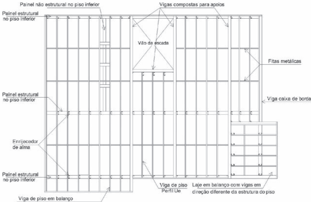
Figura 4.2 - Planta de estrutura de piso em Light Steel Framing
