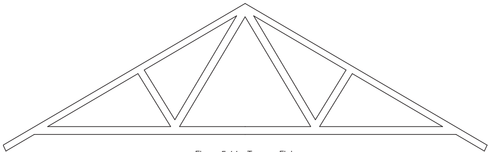
Figura 5.11 - Tesoura Fink
