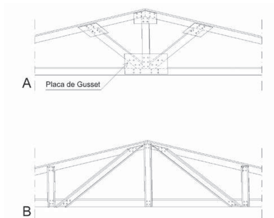
Figura 5.18 - Detalhe de cumeeira com tesoura (a) Howe e (b) Pratt
