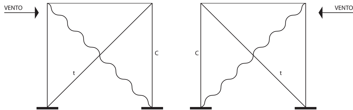
Figura 3.9 - Solicitação das diagonais de contraventamento (a partir de Dias, 1997)
