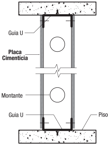
CORTE A-A FIXAÇÃO SUPERIOR E INFERIOR DA PAREDE
