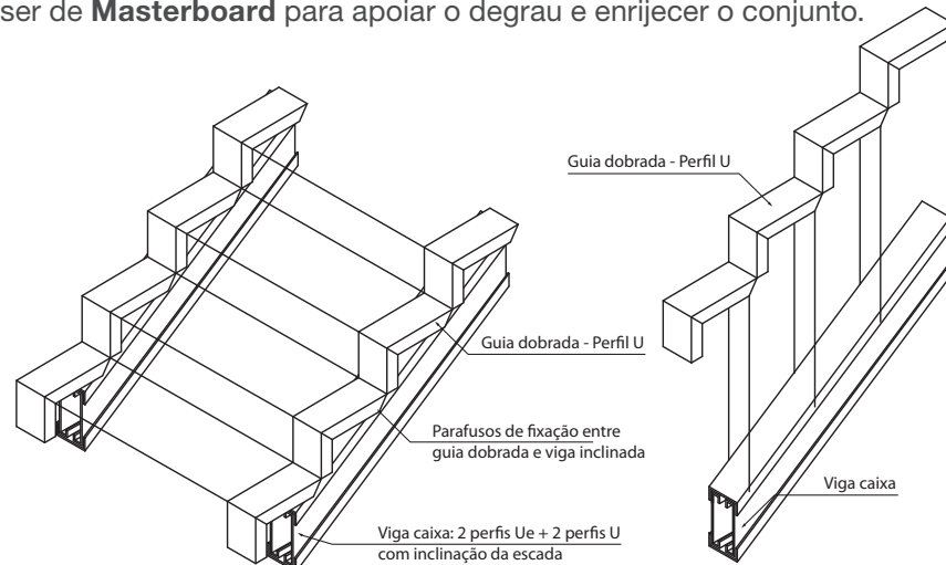
Figura 4.15 - Desenho esquemático de escada viga caixa inclinada
