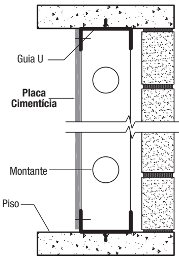
CORTE B-B REVESTIMENTO COM ESTRUTURA DE MONTANTES
