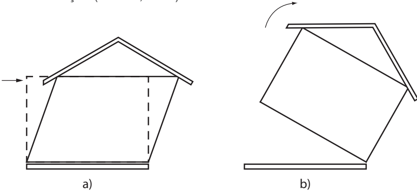
Figura 2.6 - Efeitos da carga de vento na estrutura: a) translação, b) tombamento
