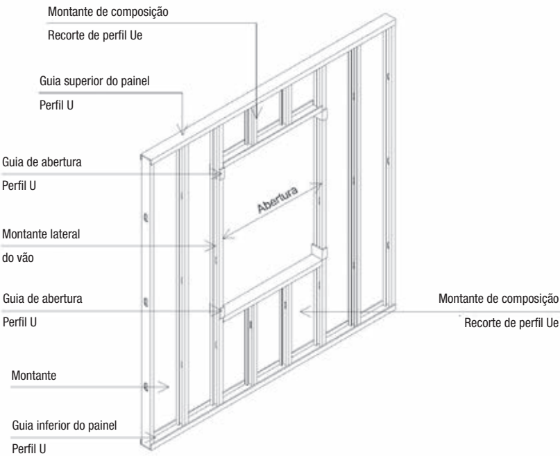
Figura 3.21 - Desenho esquemático de painel não estrutural com abertura
