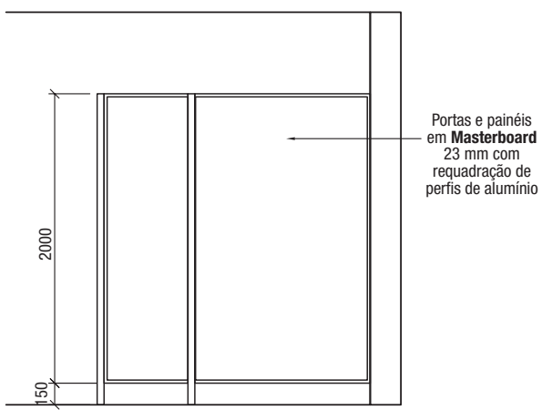
ELEVAÇÃO B
