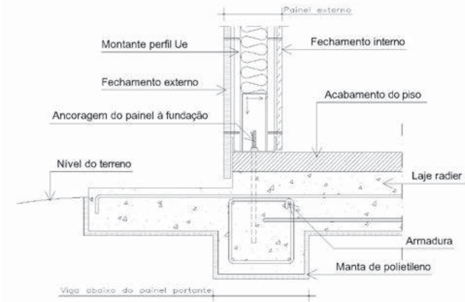
Figura 2.4 - Detalhe esquemático de ancoragem de painel estrutural a uma laje radier (adaptado de Consul Steel, 2002)
