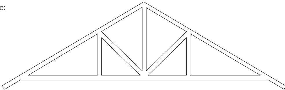
Figura 5.9 - Tesoura Howe
