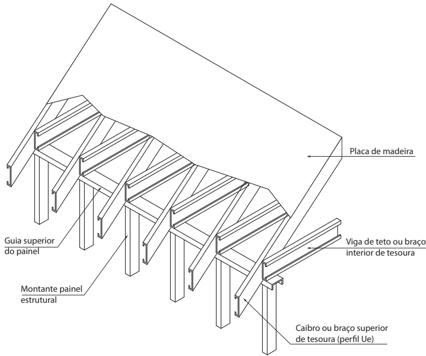
Figura 5.3 - Caibros e vigas alinhados com montantes de painel estrutural
