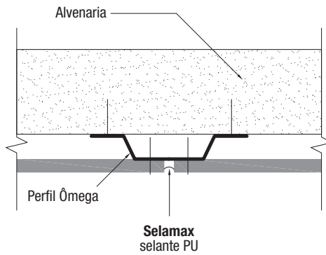
CORTE H-H
