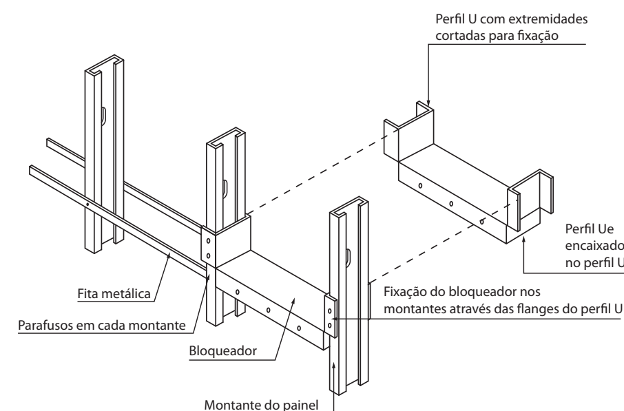
Figura 3.13 - Esquema de travamento horizontal do painel através de bloqueadores
