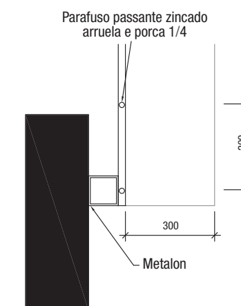
DETALHE 2
