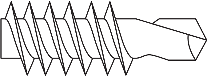
Figura 7.1 - Ponta broca
