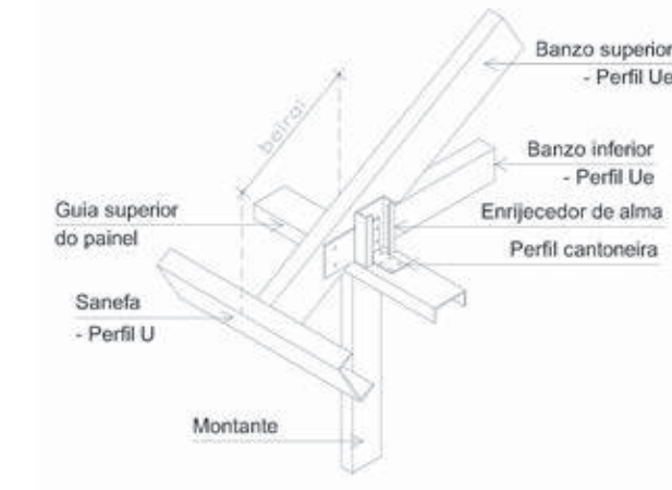
Figura 5.16 - Detalhe de beiral de telhado
