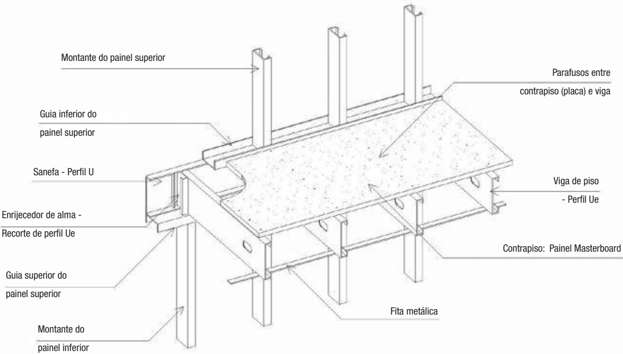
Figura 4.4 - Desenho esquemático de laje seca com pannel Masterboard
