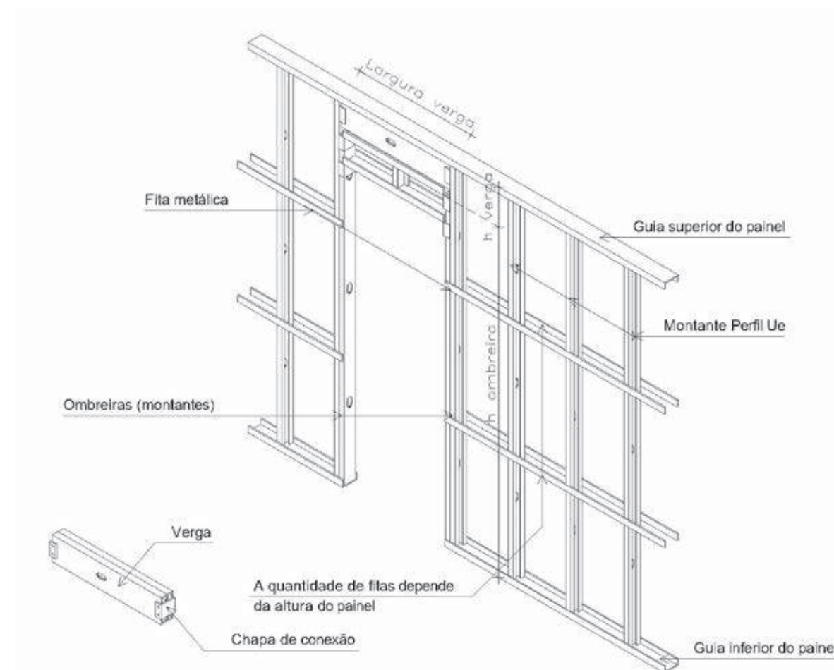
Figura 3.12 - Fita metálica para travamento de painel
