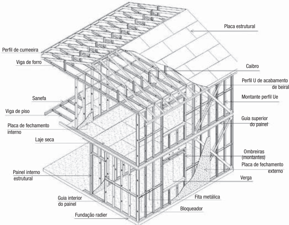
Figura 2.1 - Desenho esquemático de uma residência em Light Steel Framing
