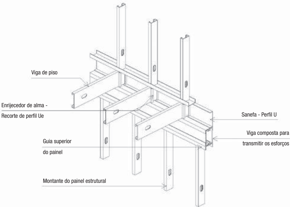
Figura 4.10 - Viga de distribuição da carga do piso para os montantes
