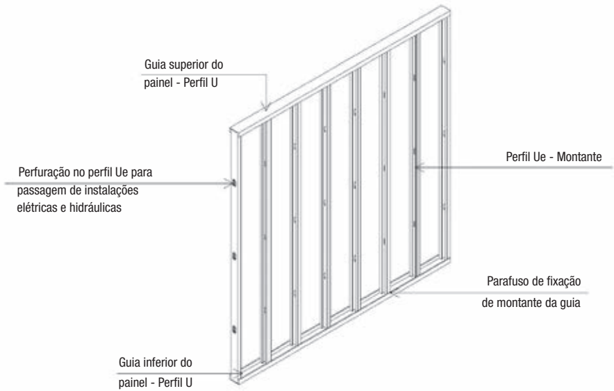
Figura 3.2 - Painel típico em Light Steel Framing
