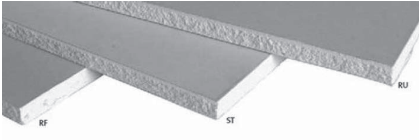
Foto 6.3 - Os três tipos de placas de gesso acartonado oferecidos no mercado (Fonte: Placo)
