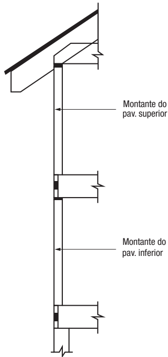
Figura 2.2 - Esquema de construção tipo “platform” (Fonte: SCI)
