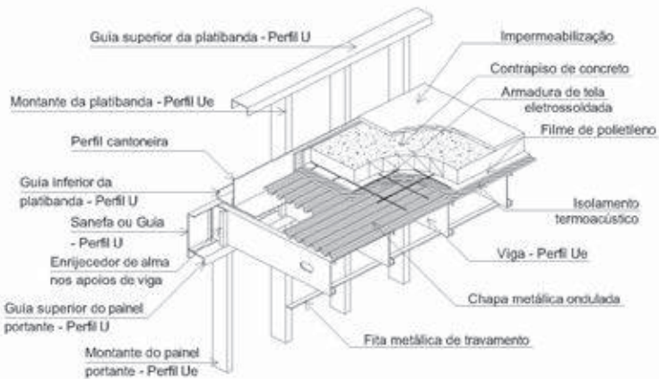
Figura 5.1 - Cobertura plana em Light Steel Framing
