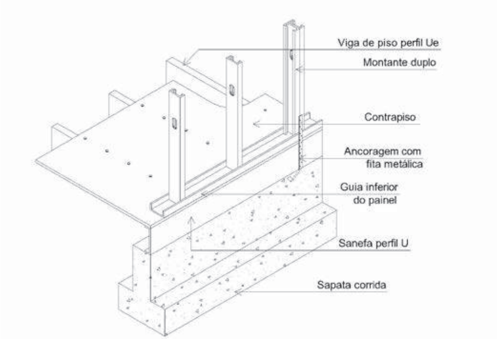
Figura 2.5 - Corte detalhado de fundação tipo sapata corrida
