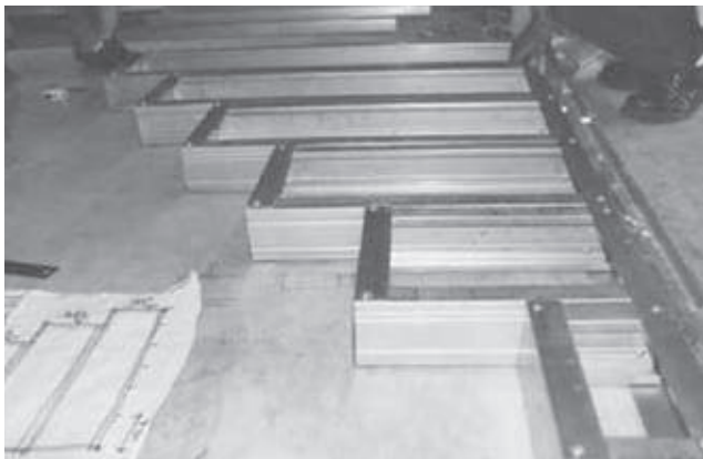
Foto 4.9 - Montagem de uma escada de painéis escalonados
