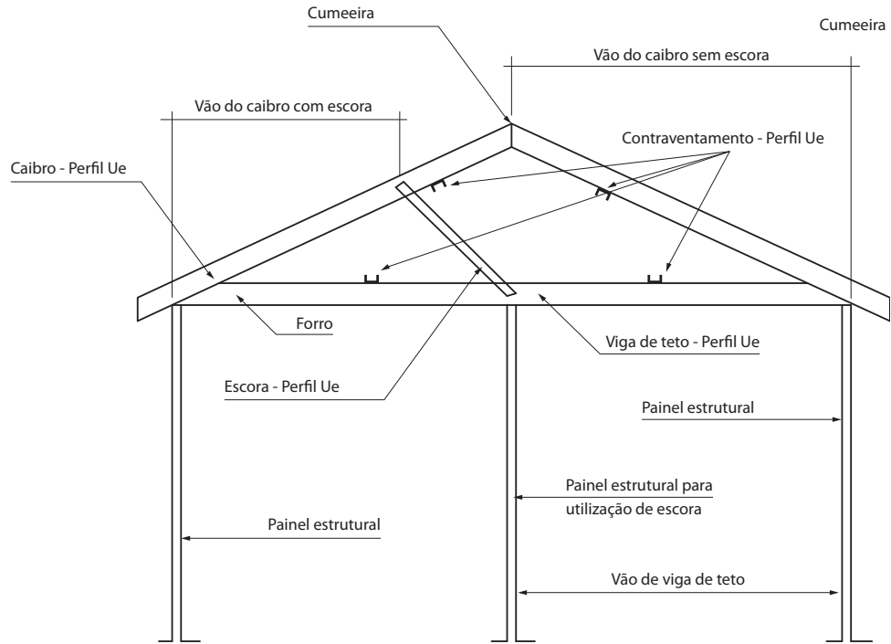
Figura 5.7 - Cobertura estruturada com caibros e vigas
