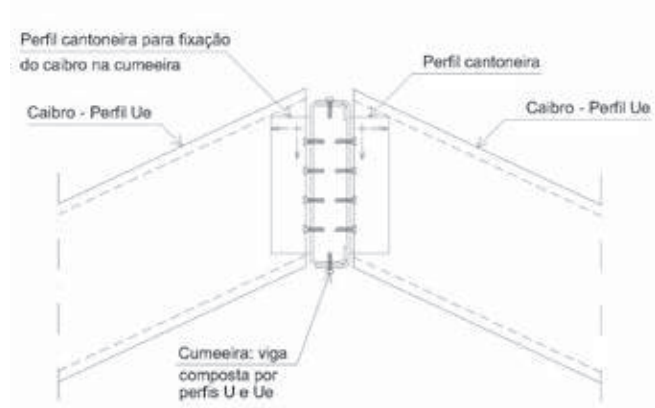
Figura 5.5 - Cumeeira de telhado estruturado com caibros
