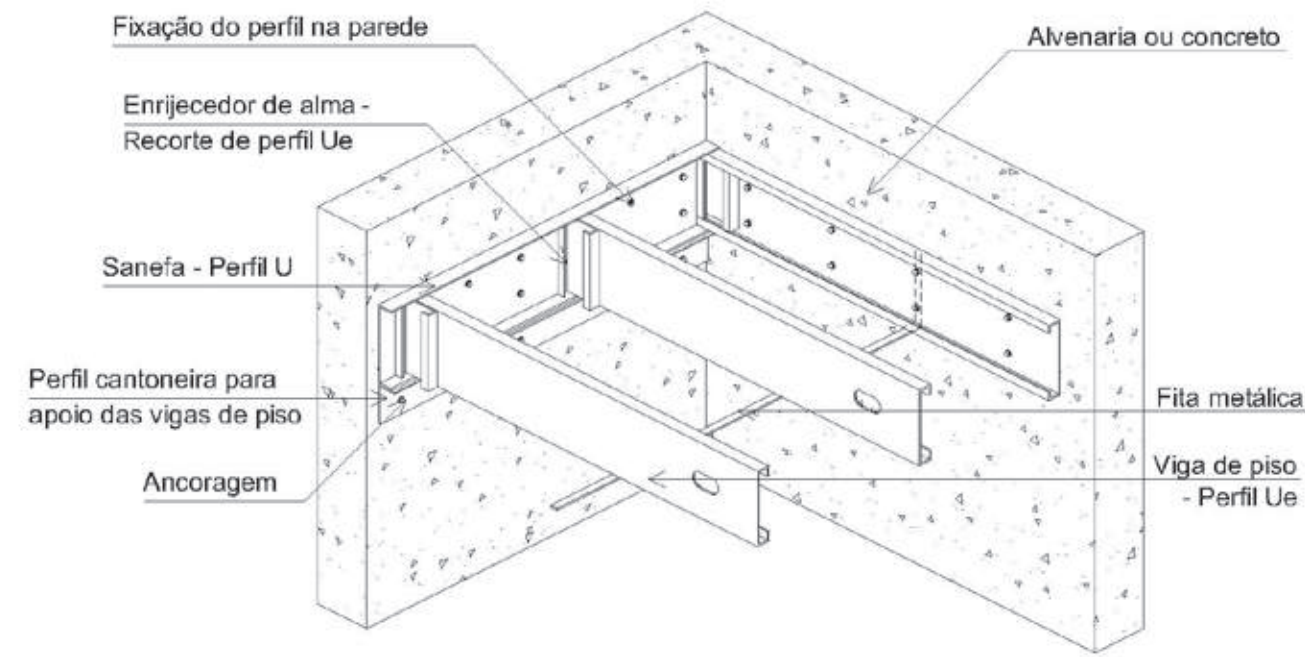
Figura 4.5 - Laje em Light Steel Framing apoiada sobre estrutura tradicional
