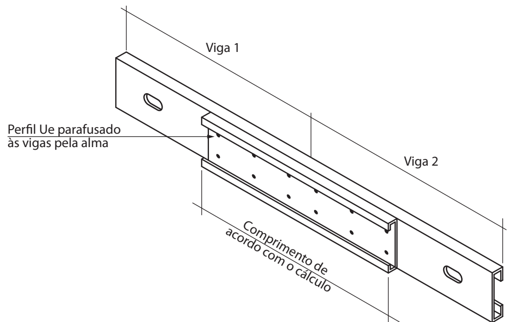
Figura 4.13 - Emenda de viga de piso
