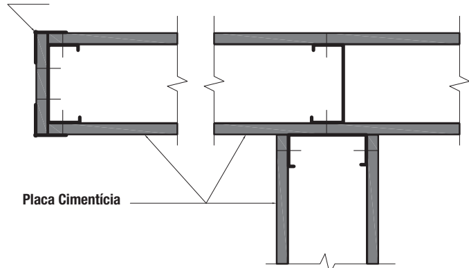
CORTE E-E ENCONTRO EM "T"
