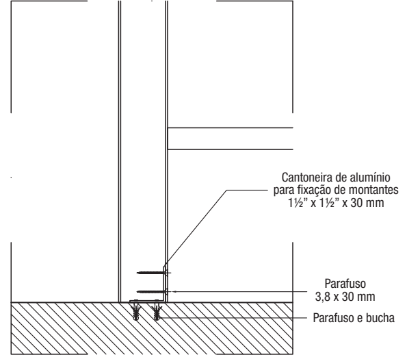
DETALHE 2
