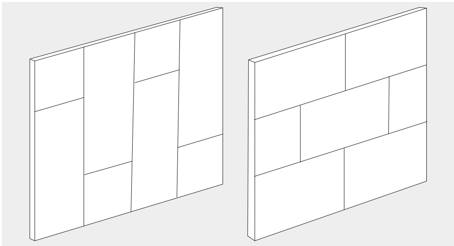
Exemplos de amarração - todas as bordas devem estar apoiadas
