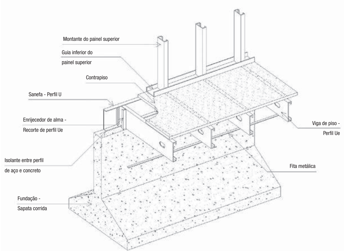
Figura 4.6 - Laje em Light Steel Framing apoiada sobre fundação tipo sapata corrida
