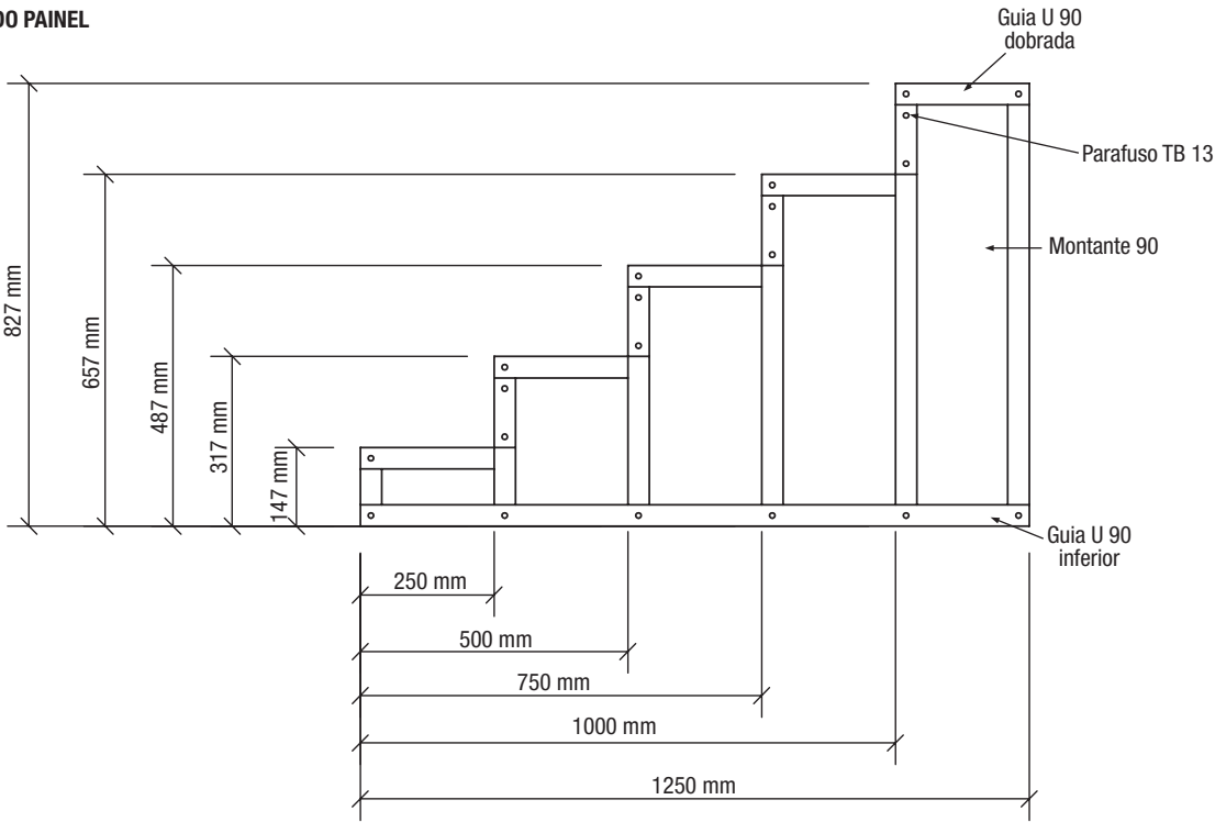
ESQUEMA DO PAINEL
