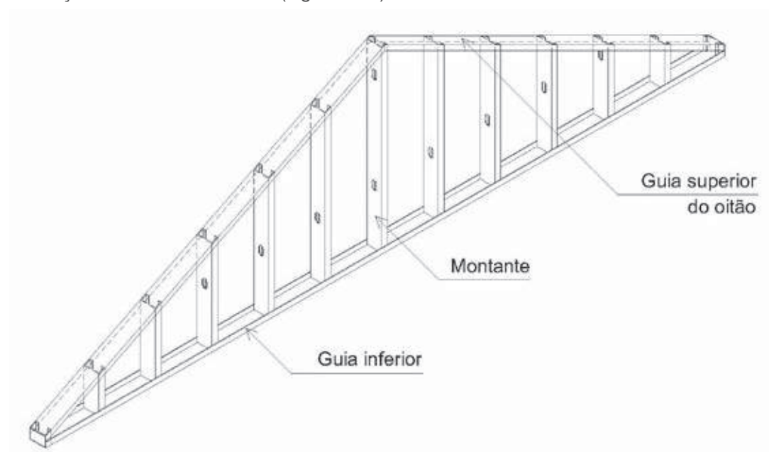
Figura 5.19 - Painel de fechamento do oitão
