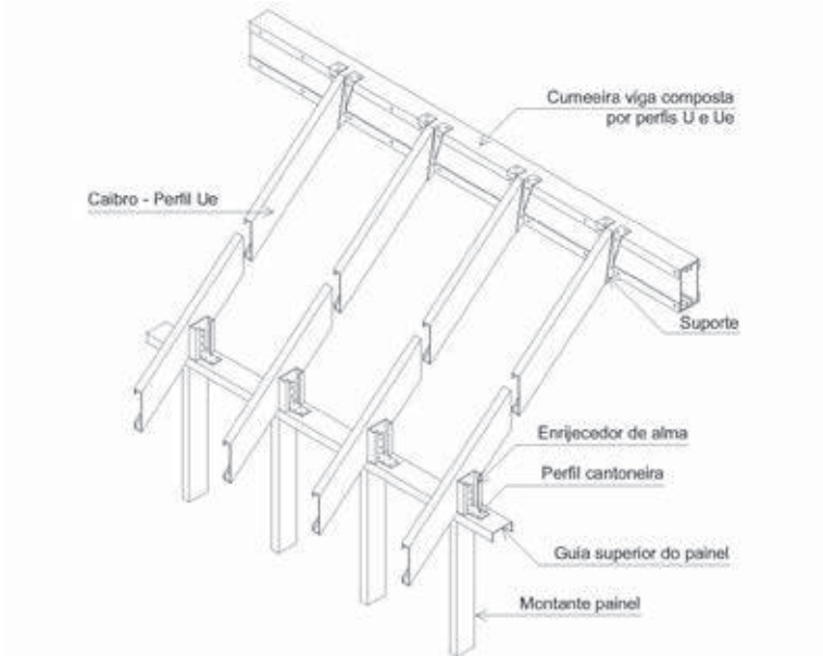
Figura 5.4 - Telhado típico estruturado com caibros
