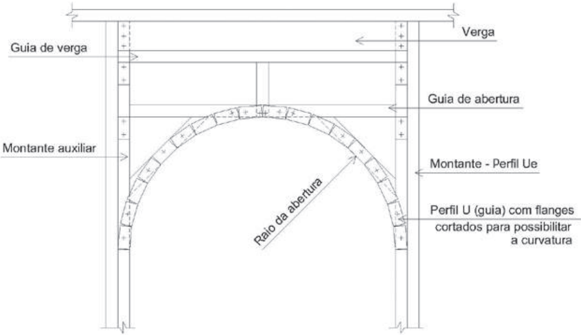
Figura 3.23 - Método para construção de aberturas em arco
