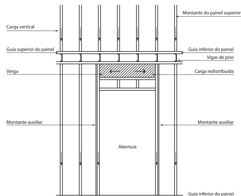
Figura 3.3 - Distribuição dos esforços através da verga para ombreiras
