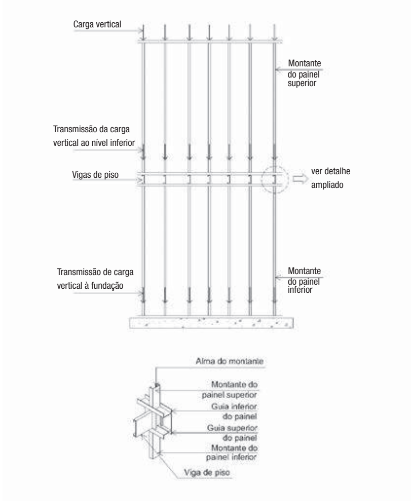
Figura 3.1 - Transmissão da carga vertical à fundação
