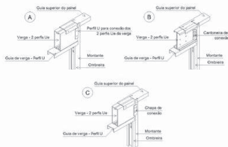
Figura 3.4 - Tipos de vergas
