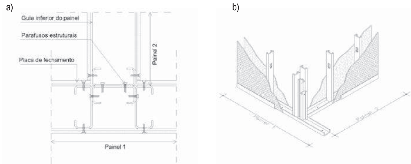
Figura 3.18 - Ligação de dois painéis formando um “T”: a) planta b) perspectiva
