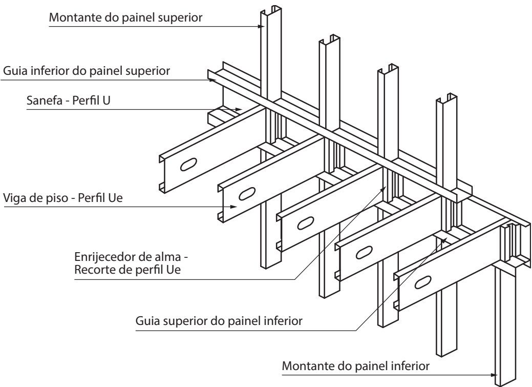
Figura 4.1 - Estrutura de piso em Light Steel Framing
