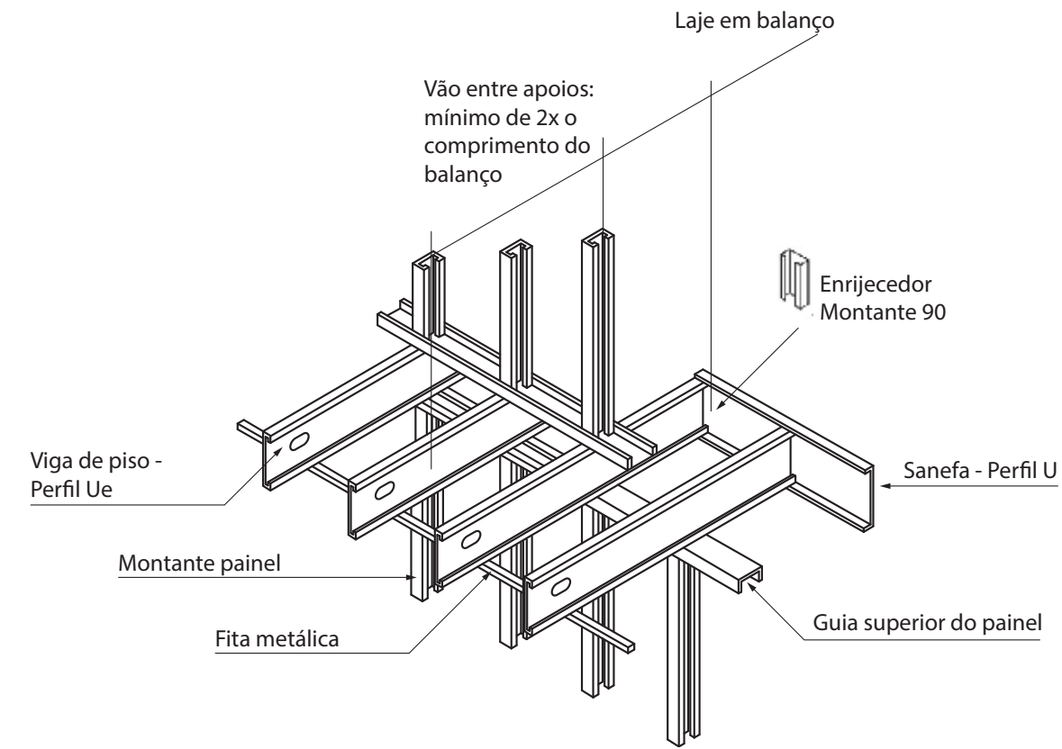
Figura 4.7 - Laje em balanço
