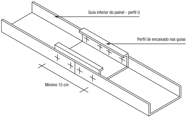
Figura 3.20 - Emenda de perfil guia
