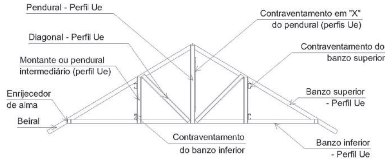
Figura 5.14 - Elementos de uma tesoura
