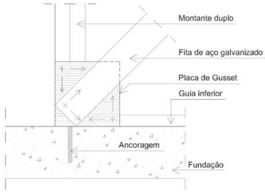
Figura 3.10 - Fixação das diagonais nos painéis por placa de Gusset
