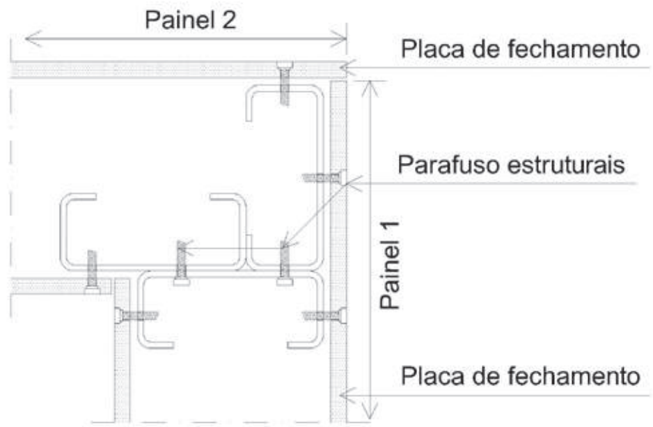
Figura 3.16 - União de três montantes
