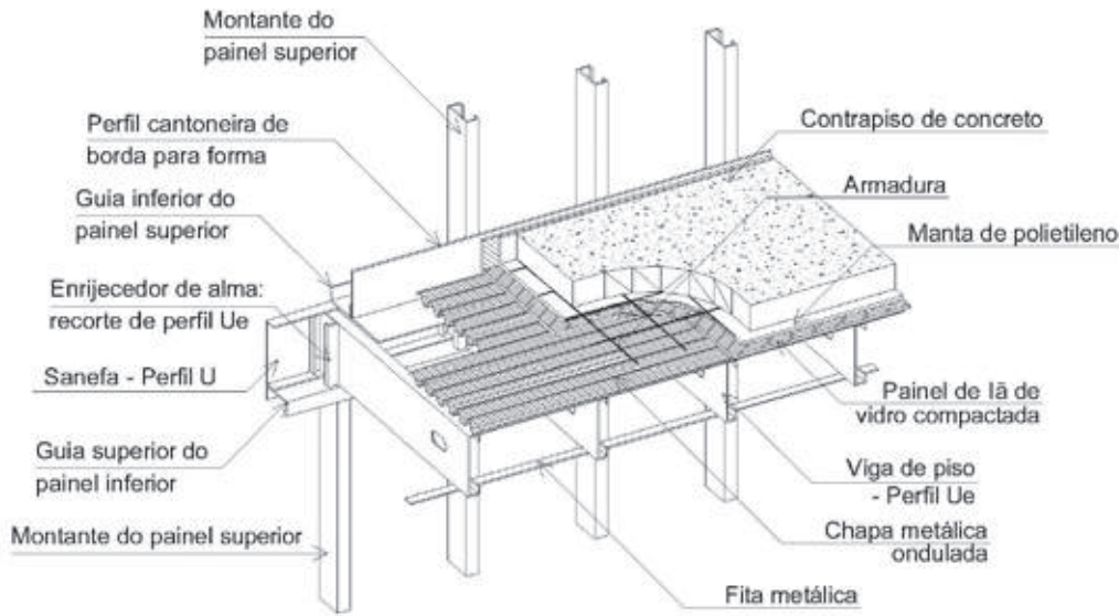
Figura 4.3 - Desenho esquemático de laje úmida
