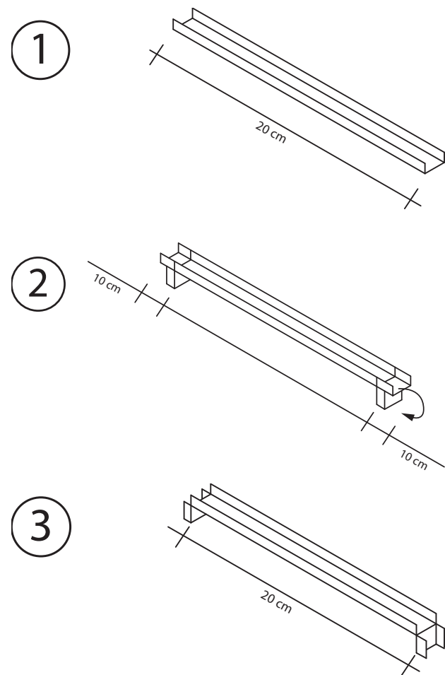
Figura 3.6 - Guia de abertura (a partir de Consul Steel, 2002)
