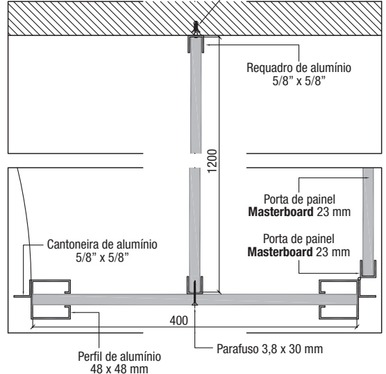
DETALHE 3
