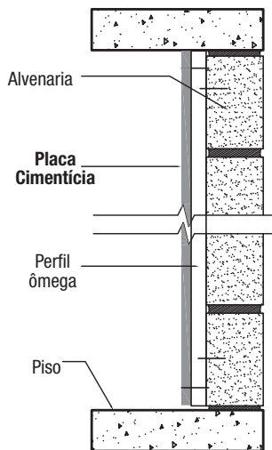
CORTE C-C REVESTIMENTO COM ESTRUTURA DE PERFIL ÔMEGA
