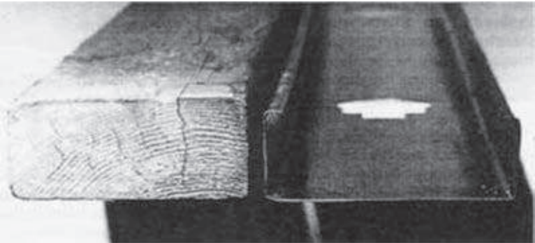
Foto 2.2 - Perfis estruturais de madeira e aço galvanizado (Fonte: Robertl Scharff)
