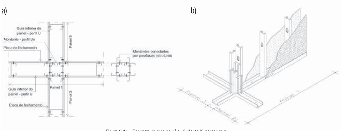
Figura 3.19 - Encontro de três painéis: a) planta b) perspectiva
