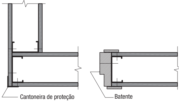
CORTE GG FIXAÇÃO DE BATENTE
