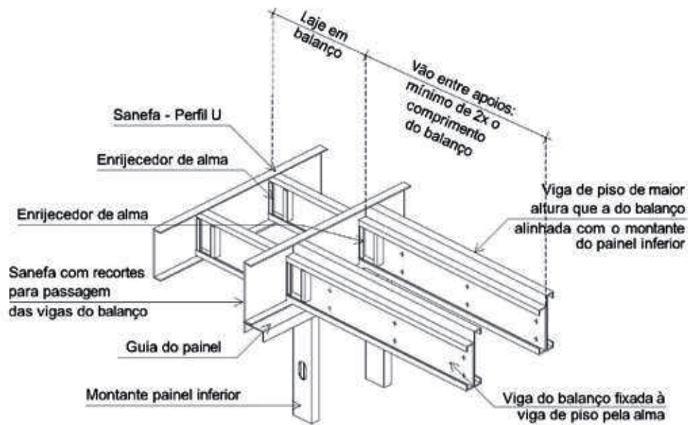
Figura 4.9 - Laje em balanço com contrapiso em níveis diferentes
