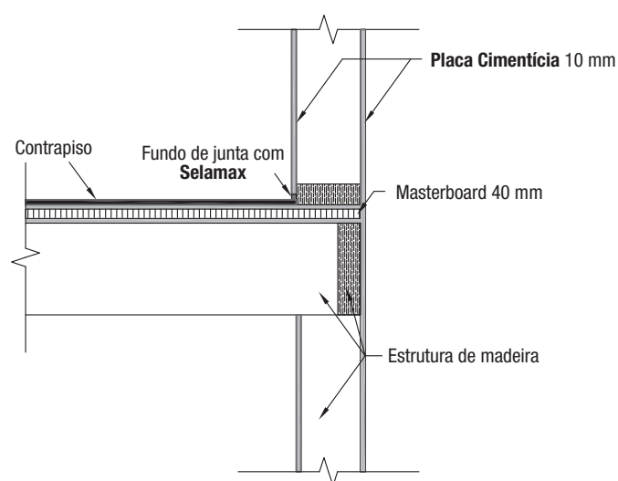
CORTE
