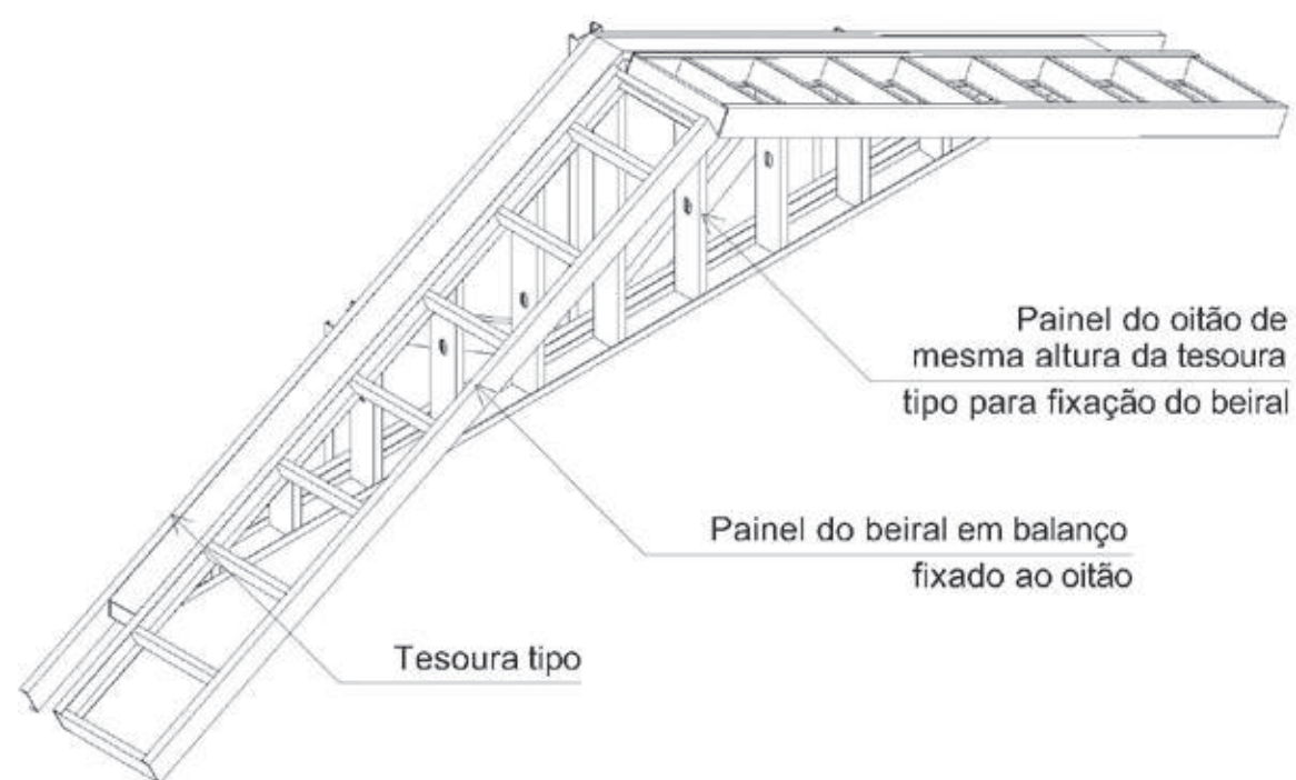
Figura 5.22 - Painel de beiral em balanço
