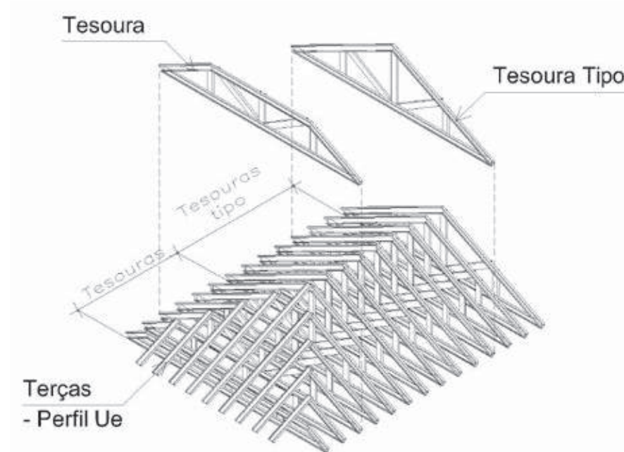
Figura 5.24 - Tesouras auxiliares
