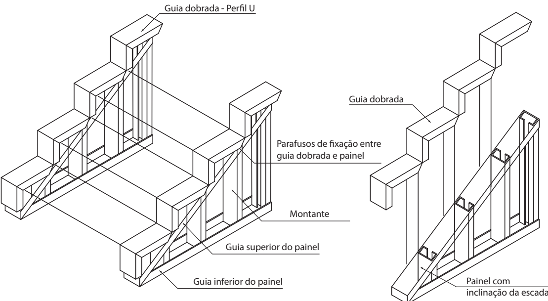
Figura 4.16 - Desenho esquemático de escada painel com inclinação
