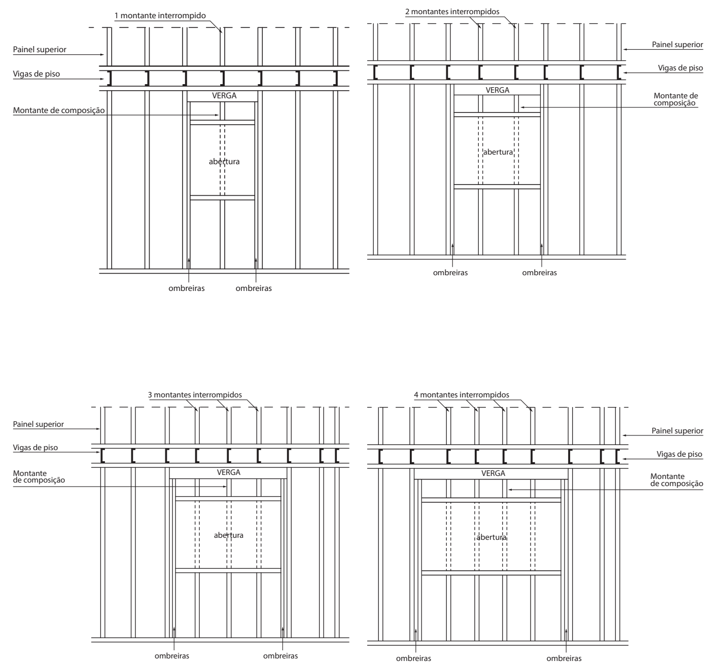
Figura 3.5 - Detalhe de ombreira
