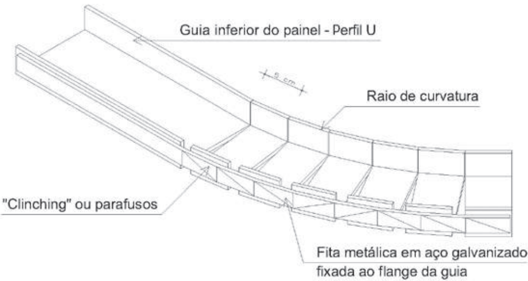
Figura 3.22 - Método para curvatura de perfis U
