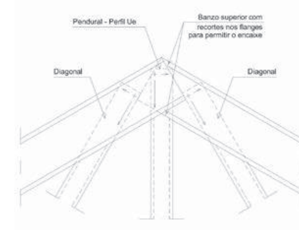
Figura 5.17 - Detalhe da cumeeira de tesoura Pratt
