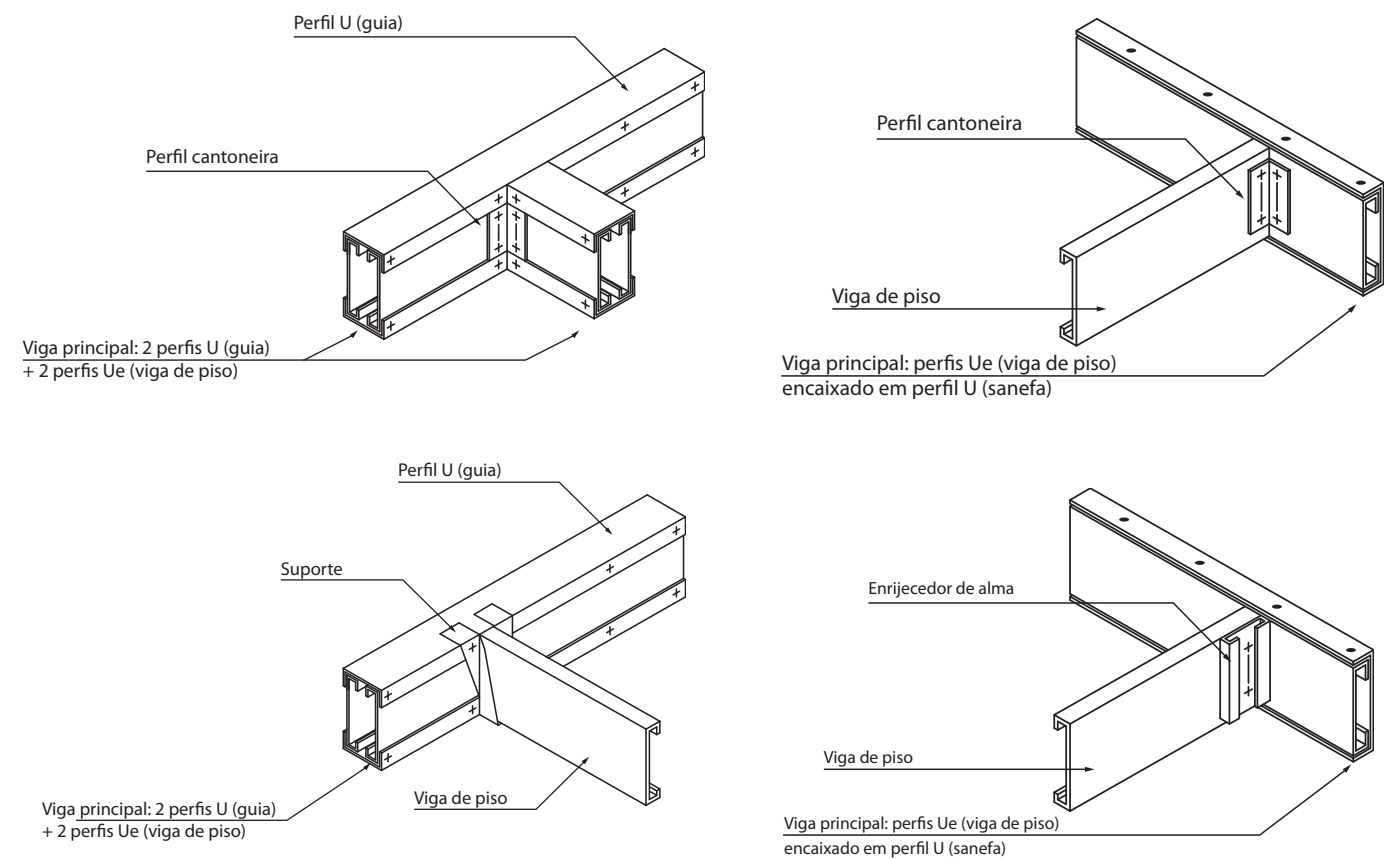
Figura 4.12 - Tipos de vigas principais para apoio de vigas de piso
