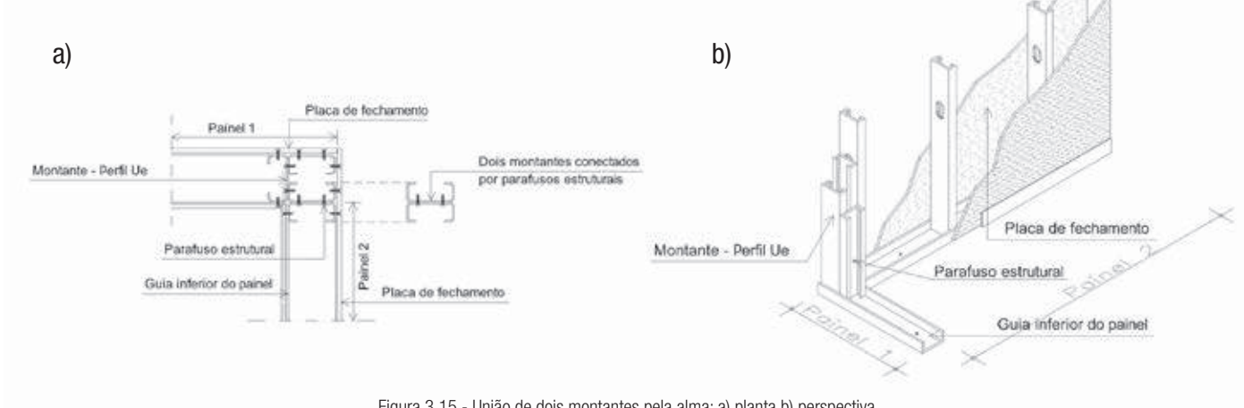
Figura 3.15 - União de dois montantes pela alma: a) planta b) perspectiva
