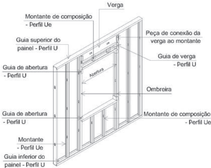
Figura 3.8 - Desenho esquemático de painel estrutural com abertura
