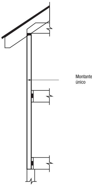
Figura 2.3 - Esquema de construção tipo “balloon” (Fonte: SCI)
