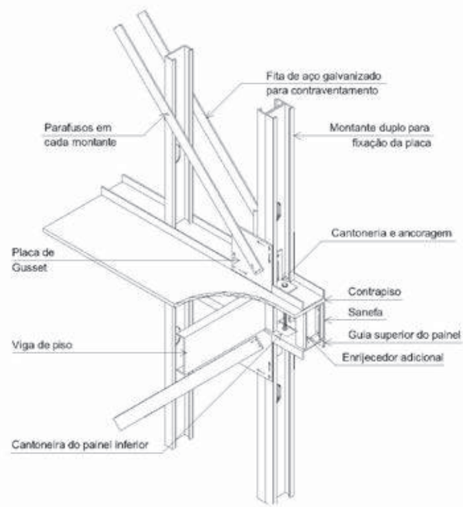
Figura 3.11 - Ancoragem de painel superior
