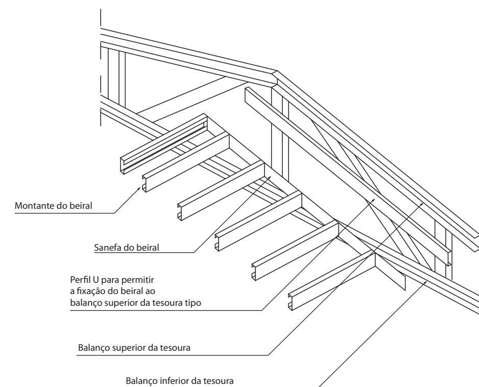
Figura 5.21 - Detalhe de fixação de painel de beiral
